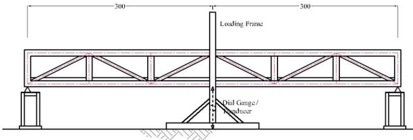
Konfigurasi Beban Tahap -2 Unit CM
