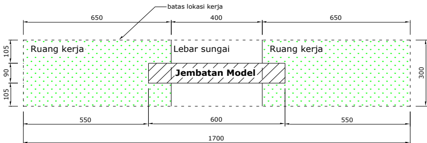
Denah Lokasi Perakitan Jembatan Unit: cm
