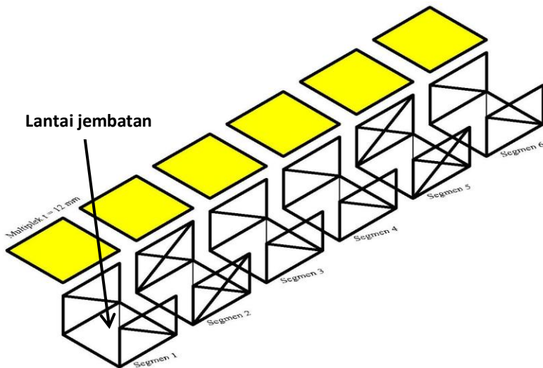
Gambar segmen Jembatan Baja
