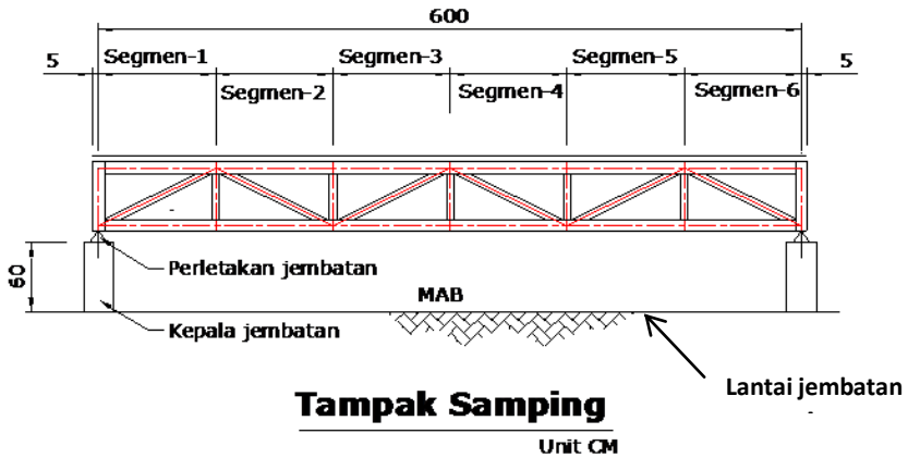
Gambar 1: BENTUK UMUM MODEL JEMBATAN BAJA
