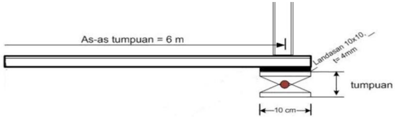
DETAIL SEGMENT 1 & 6 (Ujung Tumpuan)
