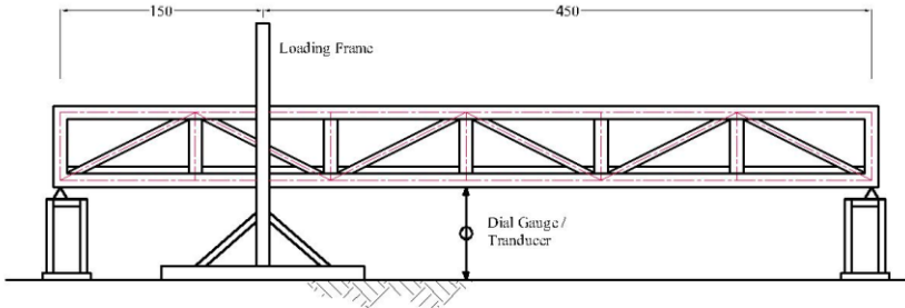
Konfigurasi Beban Tahap -1 Unit CM
